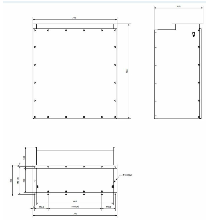
Übergangsstück OSF 1000FC / OMF 2000FC - HEPA 610x610x292mm
